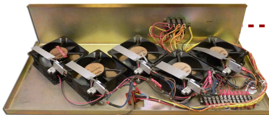
"AC" FAN TRAY
