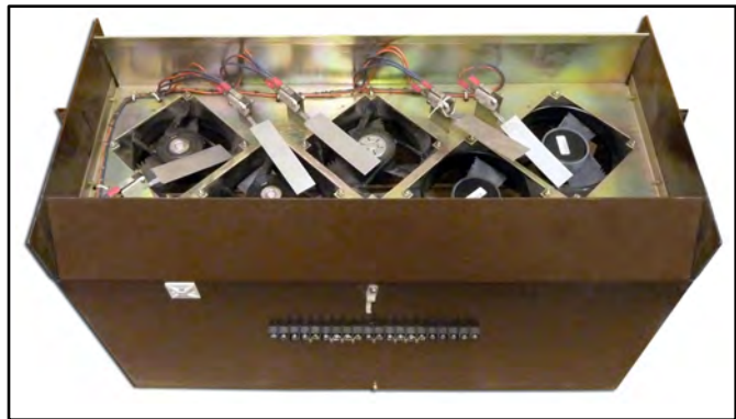
DMS-100 (NT3X90AA/AB) (AC) FAN TRAY
