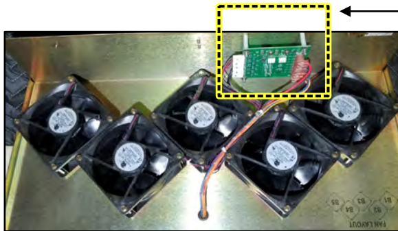
DMS-100 (NT3X90AF) FAN TRAY
