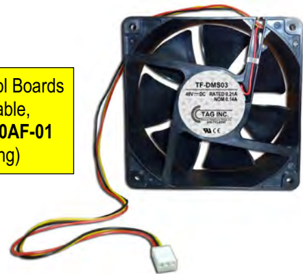
DMS-100 (NTRX91AA) FAN TRAY
